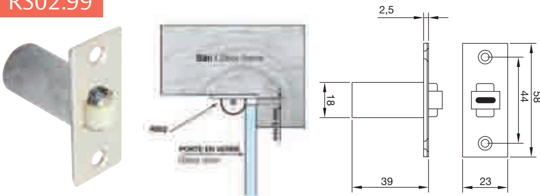
Galet avec rouleau nylon, réglable Blocking roller keep, adjustable
